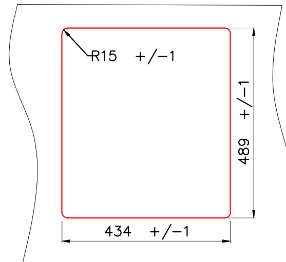
Врезной монтаж мойки (I)
