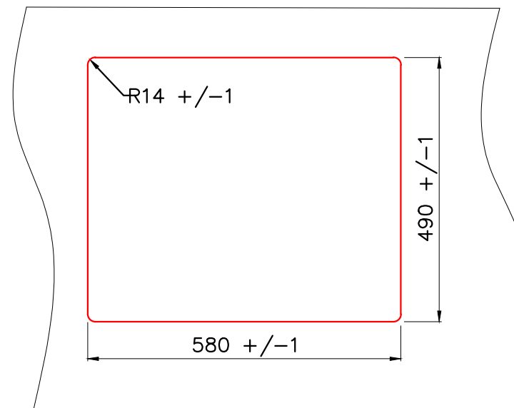
Врезной монтаж мойки (I)
